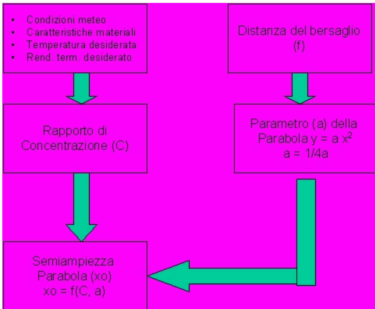
Fig. A.4.5. Schema di calcolo della distanza del bersaglio in funzione della concentrazione, delle caratteristiche materiali, della temperatura desiderata e del rendimento termico desiderato.
